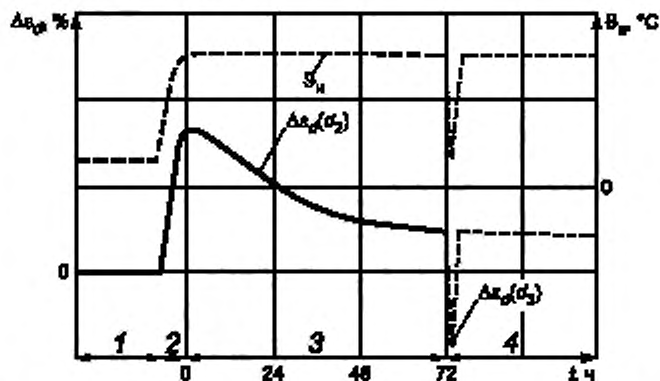
\Delta \varepsilon_d — изменение толщины, %; \theta_n — температура нагревательной пластины °C. t — время, ч. 1 — условия окружающей среды с приложением нагрузки на образец; 2 — период нагревания; 3 — период испытания; 4 — дополнительный период охлаждения и повторного нагревания (только для иллюстрации)
