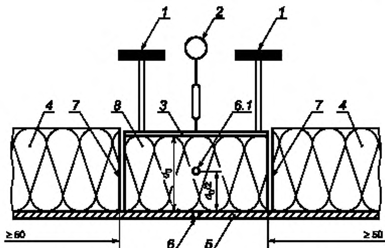
1 — винтовые упоры для задания и/или фиксации толщины образца d_0 ; 2 — прибор для измерения толщины образца (например, электромеханический); 3 — нагрузочная пластина; 4 — теплоизоляция боковых граней образца; 5 — нагревательная пластина; 6 — термопара; 6.1 — дополнительная термопара для испытаний на внутреннее самонагревание; 7 — зазор; 8 — образец
