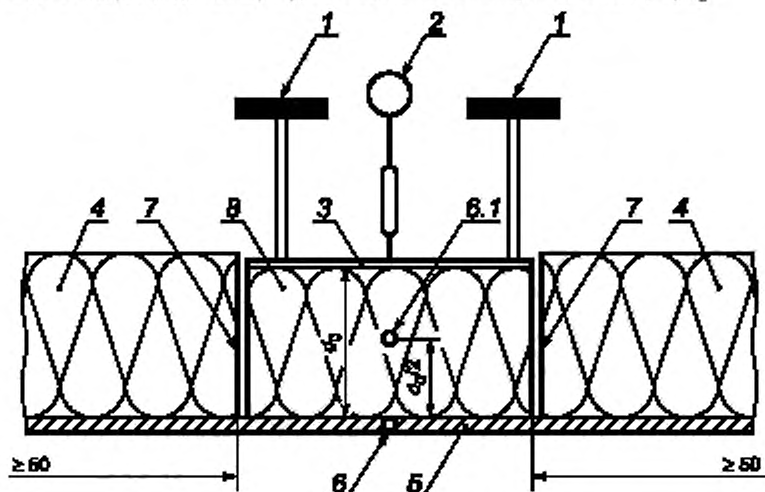
Рисунок А.1 — Схема устройства для определения максимальной рабочей температуры прошивных матов с металлической сеткой
