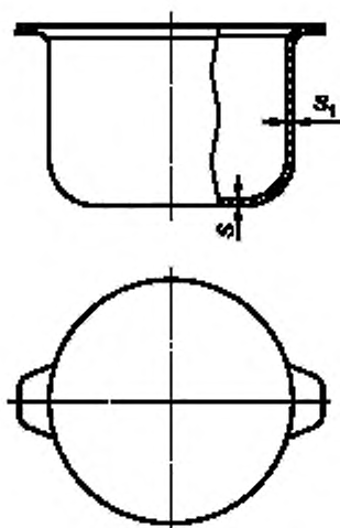
Рисунок 11 — Котел
