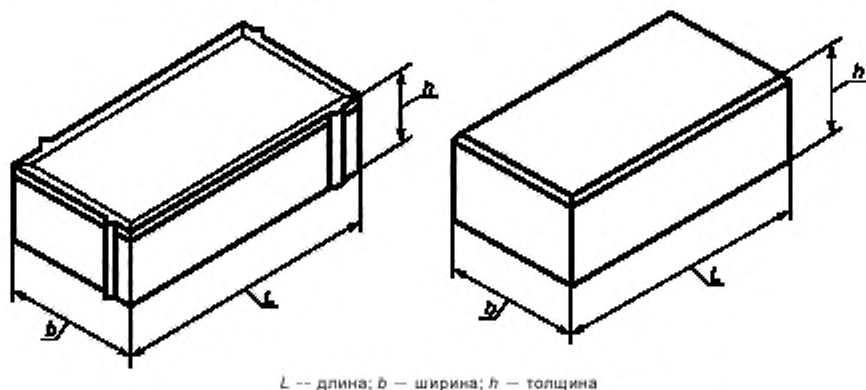
Рисунок 1 — Размеры клинкерного кирпича для мощения:
