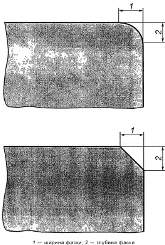
Рисунок 2 — Ширина и глубина фаски
