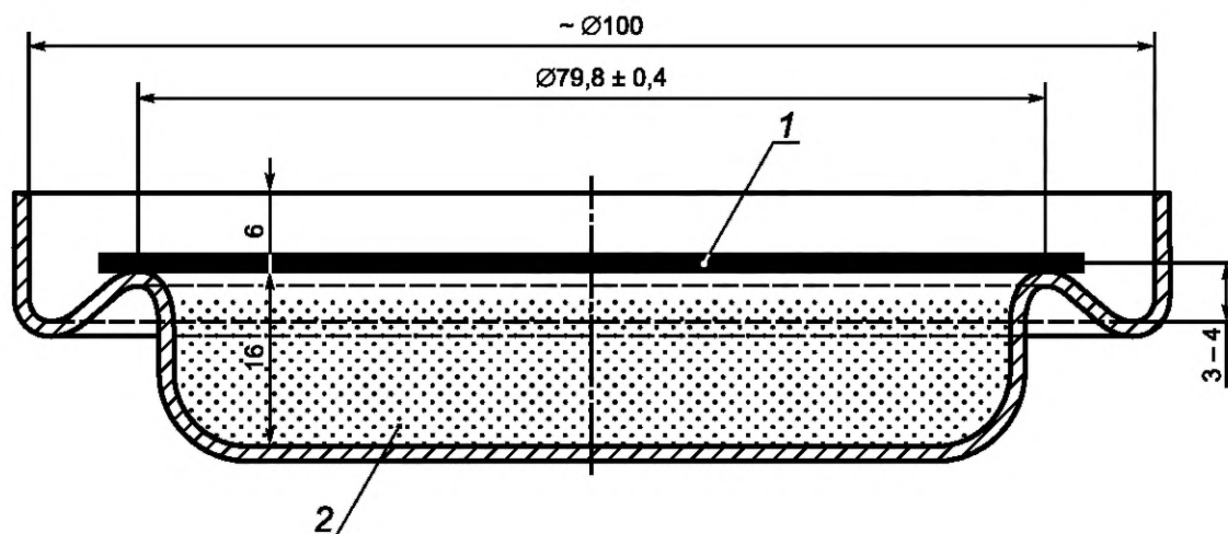
Рисунок 1 — Алюминиевая чашка с влагопоглотителем
