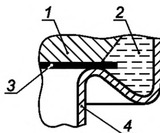
1 — шаблон; 2 — герметик; 3 — образец; 4 — чашка (см. рисунок 1)
