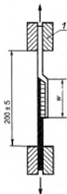
1 — зажим; w — ширина клеевого соединения
