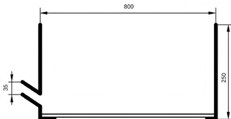
Рисунок 1 — Конструкция контейнера
