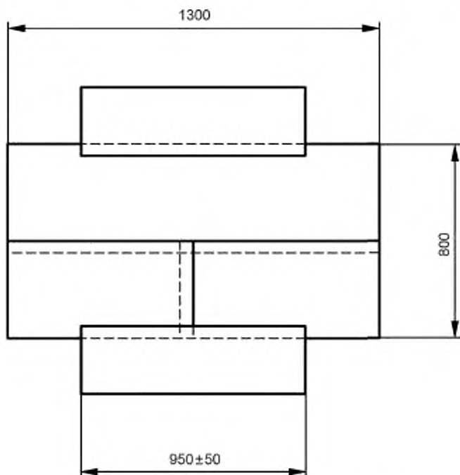
Рисунок 2 — Расположение швов в испытуемом образце
