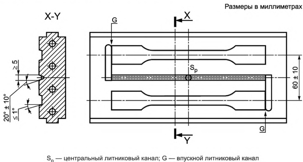
Рисунок А.1 — Схема двухгнездной литьевой формы ISO
