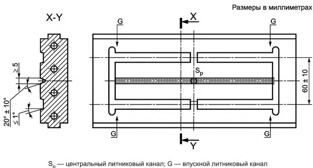
Рисунок А.2 — Схема четырехгнездной литьевой формы ISO
