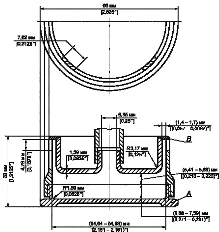
Рисунок 2 — Испарительная ячейка
