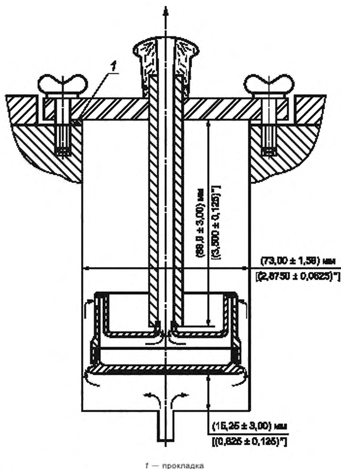
Рисунок 3 — Испарительная ячейка в сборе, помещенная в алюминиевый нагревательный блок
