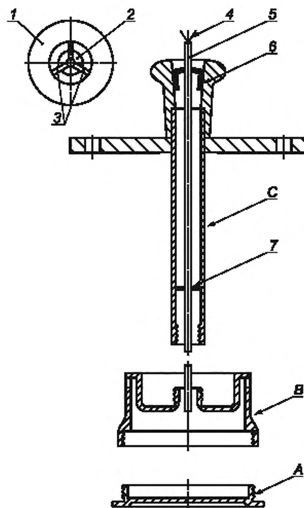
А — чашка для образца, В — колачок; С — крышка и выпускная трубка, 1 — крышка; 2, 5 — трубка для термопары; 3, 6 — подставки для термопары; 4 — термопара; 7 — стойки для центрирования термопары
