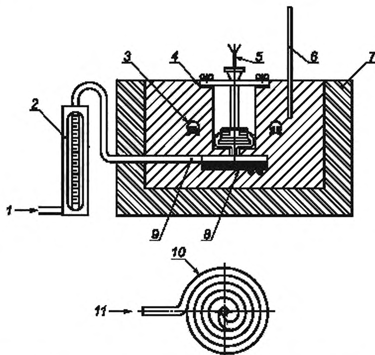
1 — подача воздуха; 2 — расходомер; 3 — патронный нагреватель; 4 — прокладка; 5 — трубка для термопары; 6 — термометр; 7 — изоляция; 8 — кольцевой нагреватель и подогреватель воздуха; 9 — подогреватель воздуха; 10 — спираль; 11 — подача воздуха
