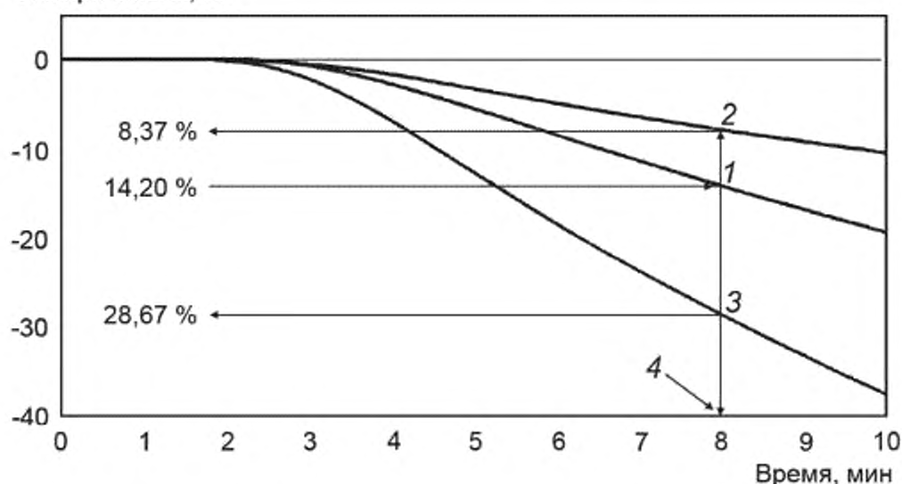
Рисунок 4 — Определение стандартного времени методом Ноак и потери от испарения испытуемых масел
