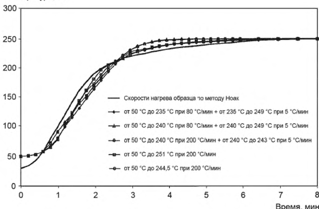
Рисунок 2 — Программы термогравиметрического анализа методом Ноак и соответствующие скорости нагрева образца
