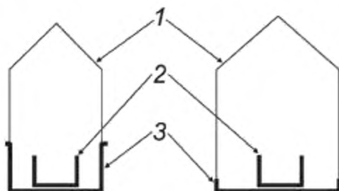
1 — проволоочная подвеска; 2 — альтернативные тигли для образцов; 3 — стандартные тигли для образцов, поставляемые в комплекте с термогравиметрическим анализатором
