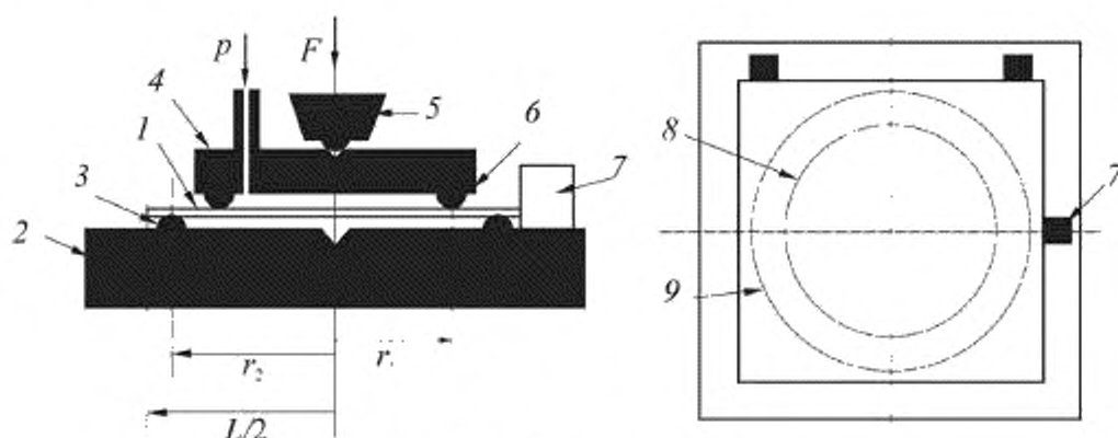
Рисунок 2 – Нагрузочное устройство
