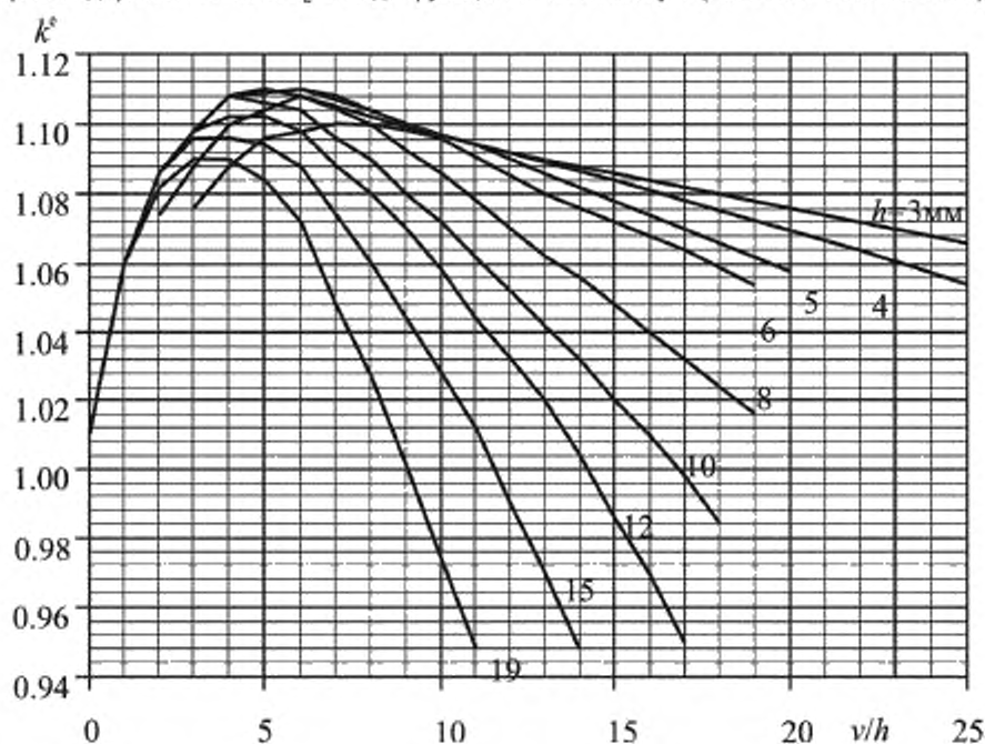
Рисунок 3 – Безразмерный коэффициент k_e как функция от y/h
