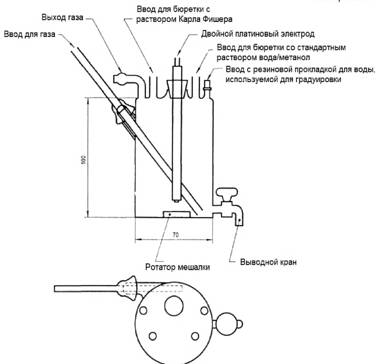
Рисунок 5 - Поглотительная ячейка
