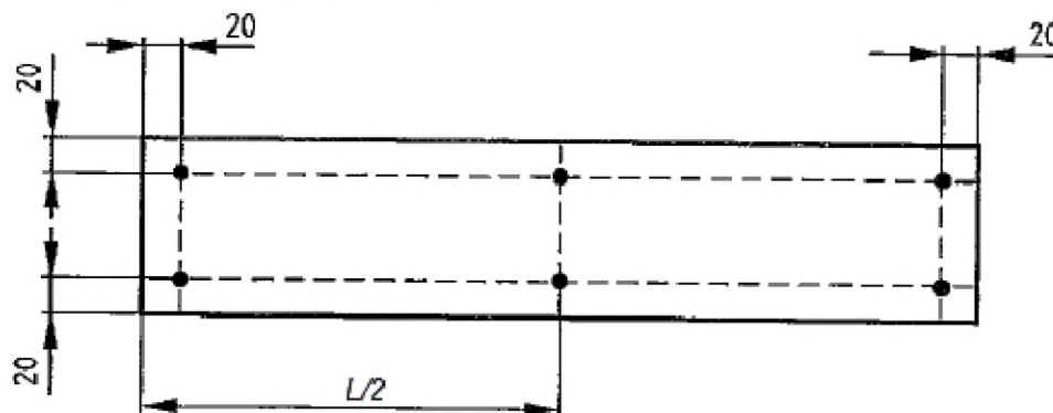
Рисунок A.3 — Точки измерения для определения толщины ( T , размеры в мм)
