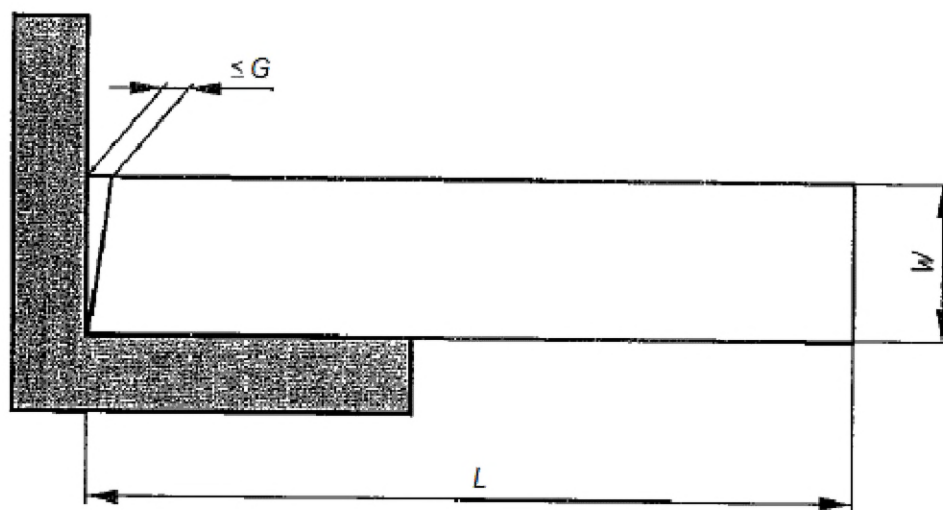
Рисунок A.4— Определение прямоугольности G
