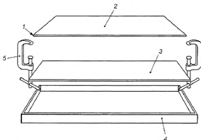
1 – пластинка для испытаний; 2 – покрытие; 3 – флот-стекло; 4 – поддон, 5 – зажим
