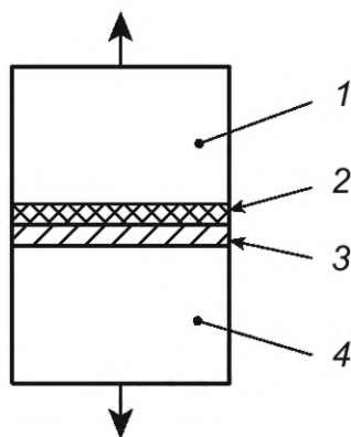
1 — окрашенная заготовка; 2 — покрытие; 3 — клей; 4 — заготовка, покрытая клеем
