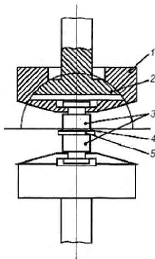
1 – опора; 2 – шаровое соединение; 3 – заготовка; 4 – лакокрасочное покрытие; 5 – окрашиваемая поверхность
