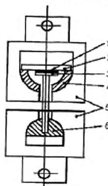
1 – лакокрасочное покрытие; 2 – окрашиваемая поверхность; 3 – заготовка; 4, 6 – шаровой подвижный шарнир; 5 – опора (сконструированная под соединение в сборе)
