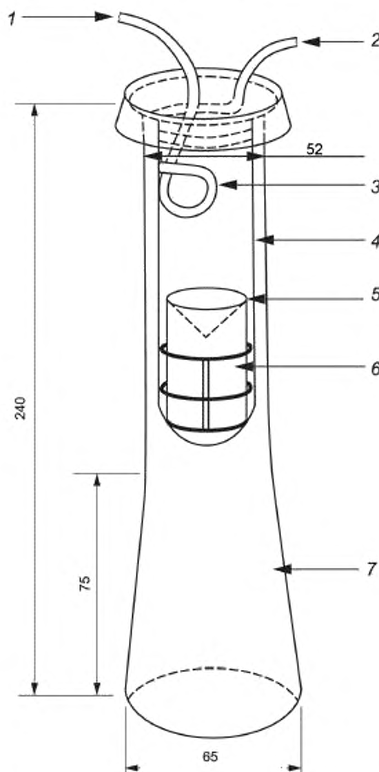
1 — вход воды; 2 — выход воды; 3 — металлический холодильник; 4 — проволочная опора, закрепленная на крючке на верхней части холодильника; 5 — бумажный конус; 6 — алундовый стакан; 7 — колба
