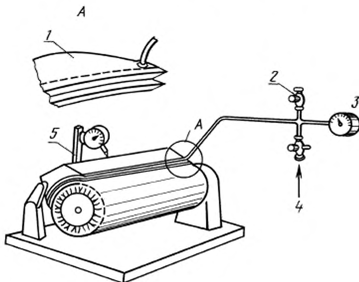
1 — подушка; 2 — выходной клапан воздуха; 3 — манометр; 4 — сжатый воздух; 5 — приспособление для измерения расстояния
