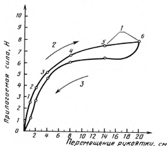
1 — точки измерения; 2 — открытый цикл; 3 — закрытый цикл
