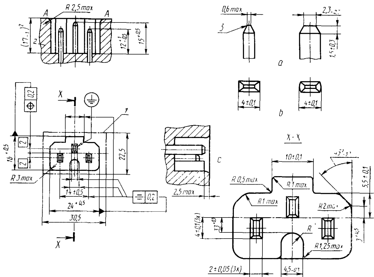
a — варианты исполнения конца штырей; b — варианты формы штырей; c — деталь направляющего элемента
