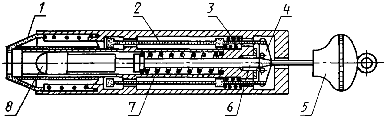
1 — вытягивающий конус; 2 — закрепляющий стержень; 3 — пружина закрепляющего механизма; 4 — зажим; 5 — кнопка управления; 6 — стержень ударяющей детали; 7 — пружина ударяющей детали; 8 — головка молотка
