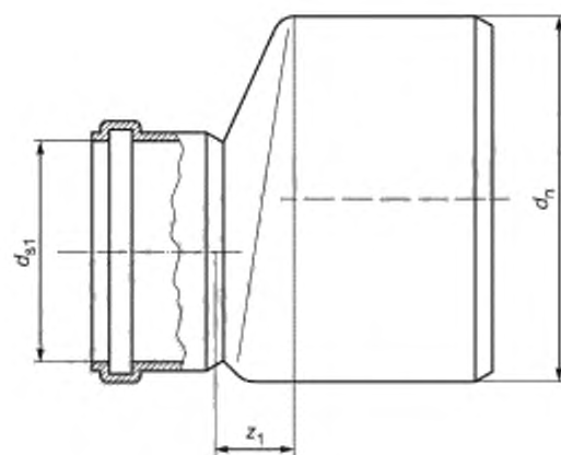
Рисунок 7 — Патрубок переходной
