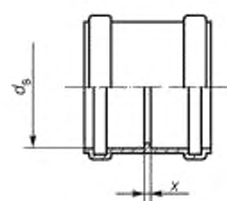
а) муфта (двухраструбная)
