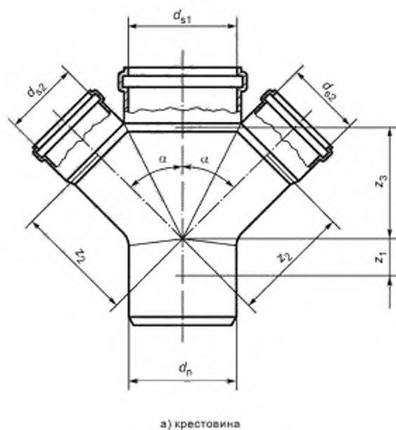
Рисунок 6 — Крестовина
