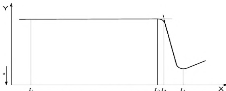
Рисунок 4 — Типичная кривая ДСК при определении термостабильности
