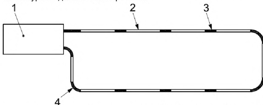
1 – ротационный насос и система нагрева; 2 – отрезки труб из PVC-C тип I длиной 300 мм; 3 – муфта PVC-C тип I; 4 – угольник PVC-C тип I
