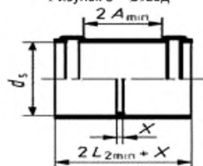
Рисунок 7 — Муфта
