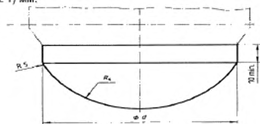
Рисунок 12 – Боек падающего груза
