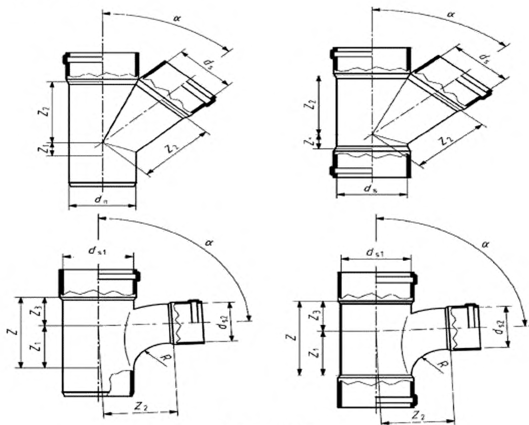
Рисунок 9 – Тройник
