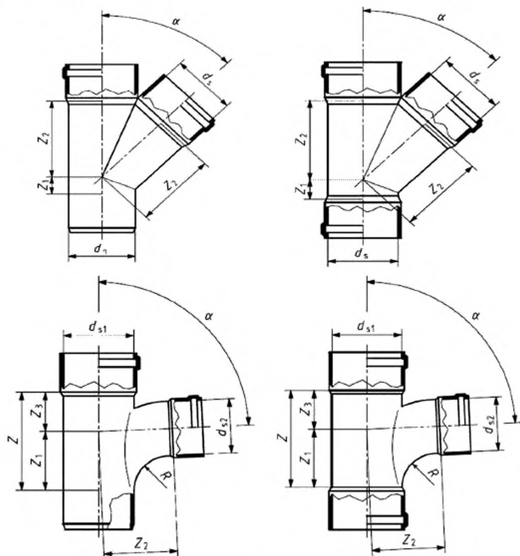
Рисунок 9 – Тройник
