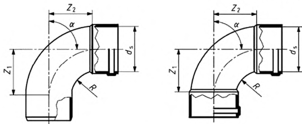
Рисунок 6 – Отвод
