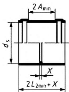
Рисунок 7 – Муфта
