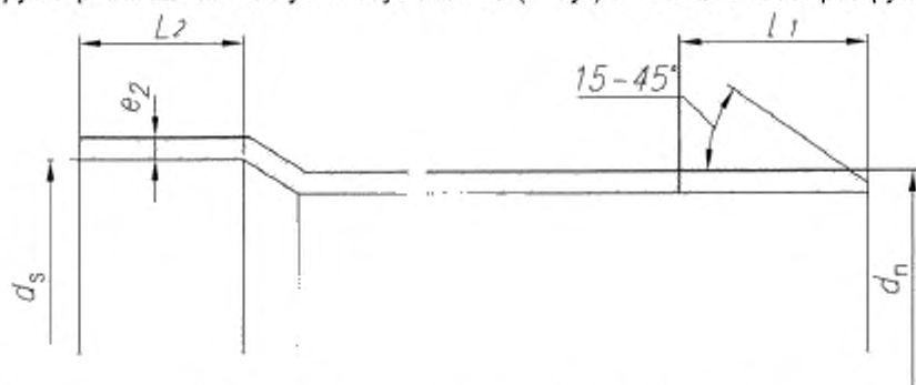
d_{\text{с}} – внутренний диаметр раструба; L_1 – длина трубного конца; L_2 – длина раструба; e_2 – толщина стенки раструба
