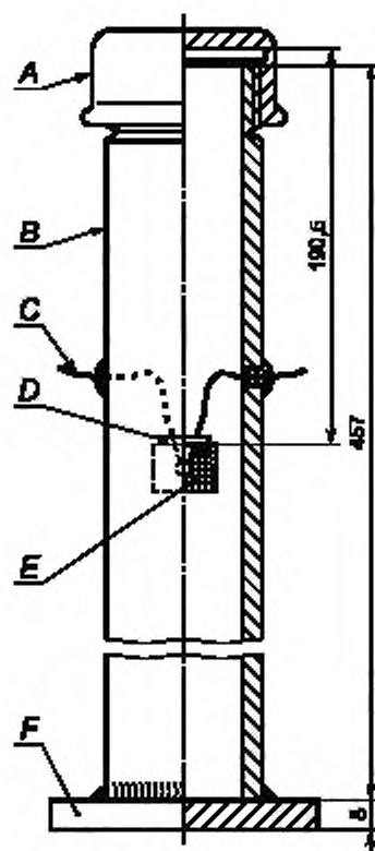
А — кованный стальной колпак, В — стальная труба; С — выводы воспламенителя; D — уплотнение, Е — комплект воспламенителя; F — контрольная плита
