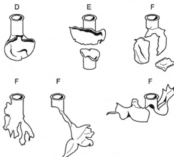
Рисунок 6 — Примеры разрушений видов D, E и F
