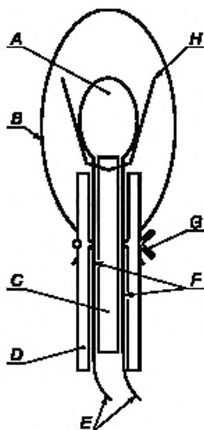
А — мостик накалывания; В — пленка из поливинилхлорида; С — изоляция; D — трубка из кремнийорганического каучука; E — запальные выводы; F — контакты из фольги; G — проволока для водонепроницаемой герметизации; H — запальный кембрик
