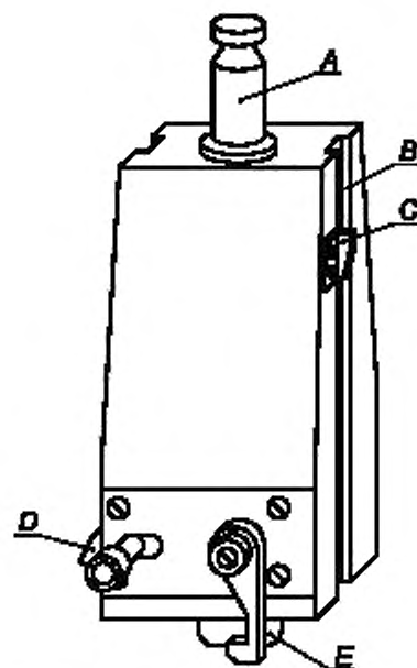
А — стержень подвески; В — направляющий паз; С — отметка высоты; D — стопор отскока; Е — цилиндрическая ударная головка
