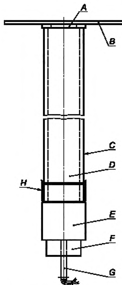
А — прокладки, В — контрольная пластина, С — стальная трубка; D — испытуемая химическая продукция; E — бустер, состоящий из циклотриметилнитрида/парафина или ТЭН/тротила; F — держатель детонатора; G — детонатор; H — пластмассовая мембрана
