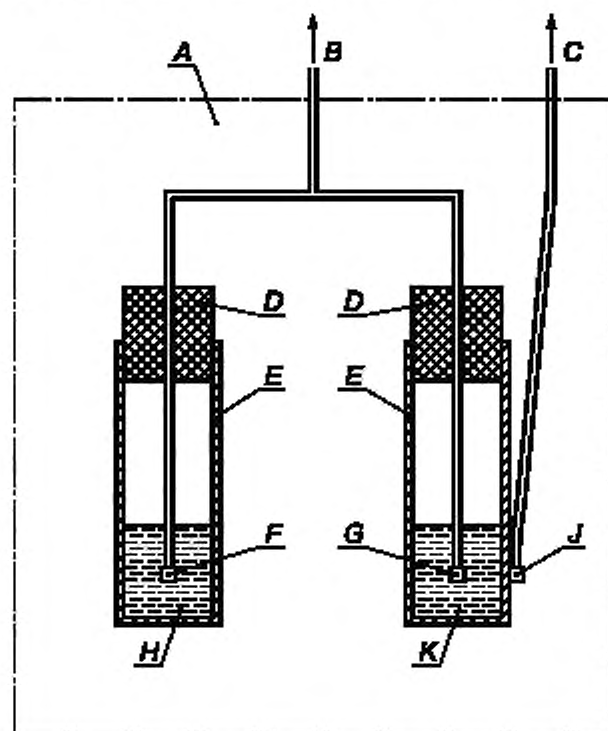
A — печь. B — к милливольтметру ( T_1 - T_2 ); C — к милливольтметру ( T_3 ); D — пробирка, E — пробирка; F — термопара № 1 ( T_1 ), G — термопара № 2 ( T_2 ); H — 100 см 3 образца; J — термопара № 3 ( T_3 ); K — 100 см 3 эталонной химической продукции
