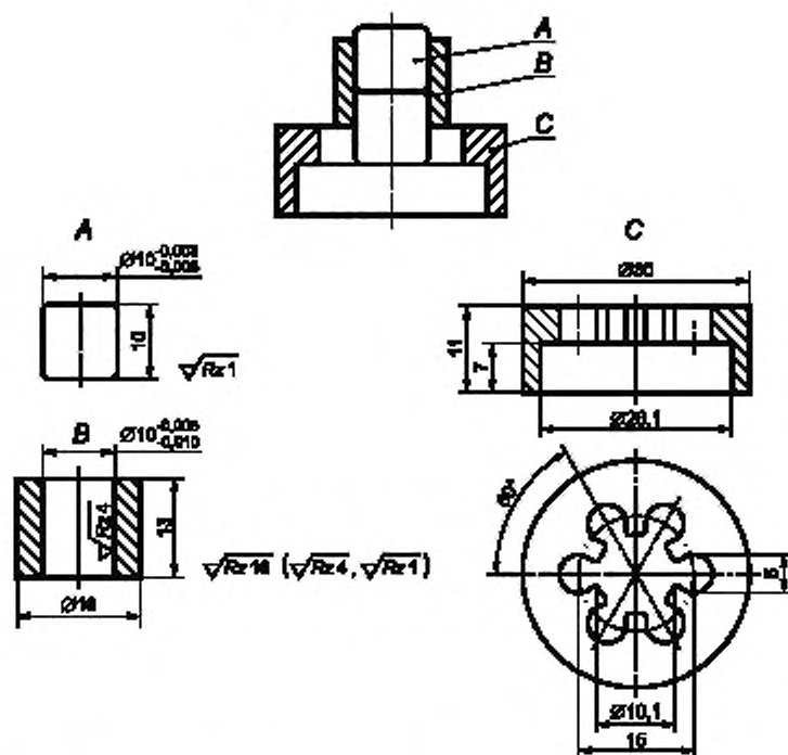
А — стальной(ые) цилиндр(ы); В — направляющее кольцо; С — центрирующее кольцо
