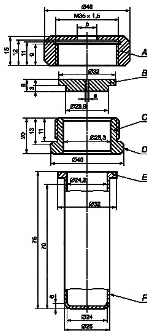
А — гайка ( b = 10,0 или 20,0 мм), рассчитанная на гаечный ключ 41; В — пластина с отверстием ( a = 1,0 \cdot 20,0 мм в диаметре); С — резьбовое кольцо; D — фаски для гаечного ключа 36; E — фланец; F — трубка
