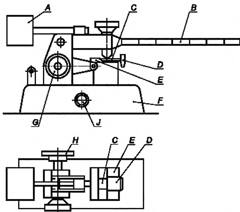
А — противовес; В — плечо для груза; С — фарфоровая пластина, прикрепленная к каретке; D — регулятор; E — подвижная каретка; F — стальная опора; G — рычаг для приведения каретки в начальное положение; H — указатель направления к электромотору; J — выключатель
