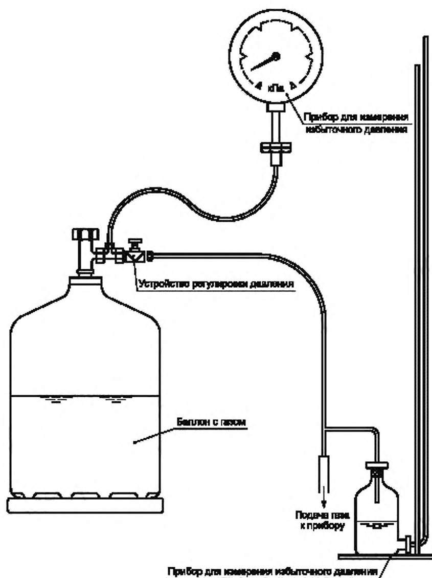
Рисунок 1 — Аппаратура для измерения повышения давления
