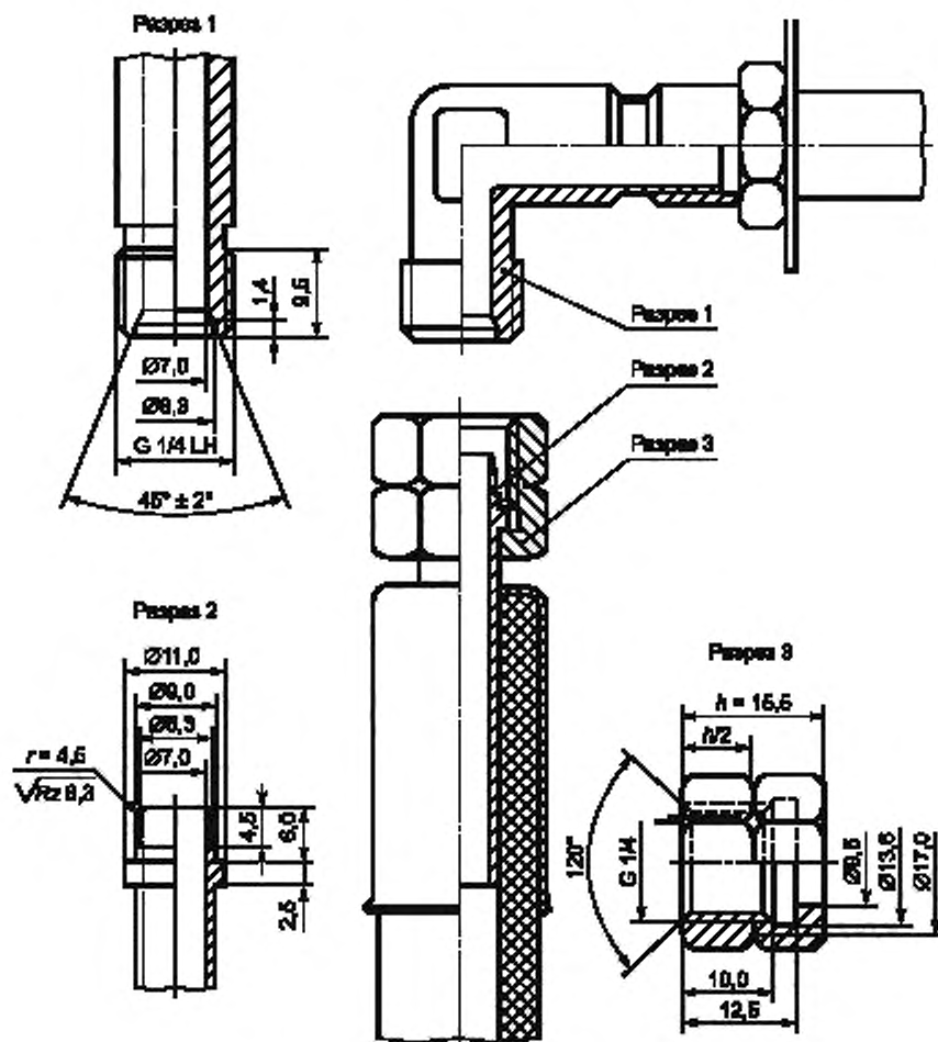
Рисунок Б.1 — Муфты для шлангов
