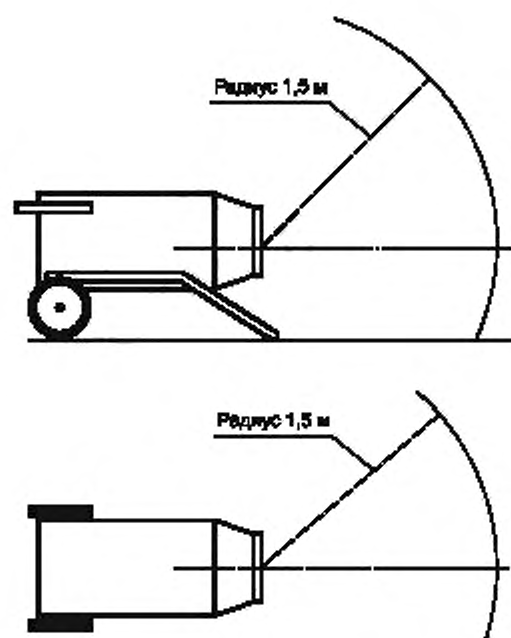
Рисунок 2 — Измерение температуры нагнетаемого воздуха
