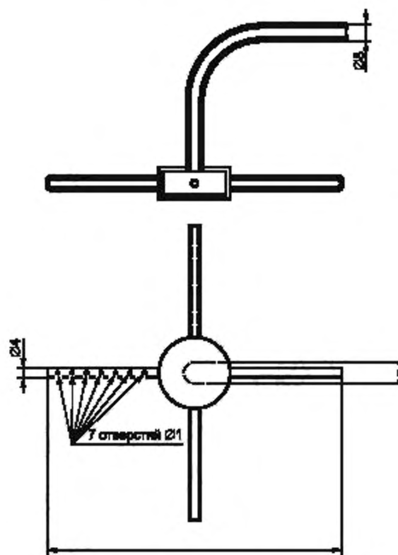
Рисунок 3 — Пробоотборник
