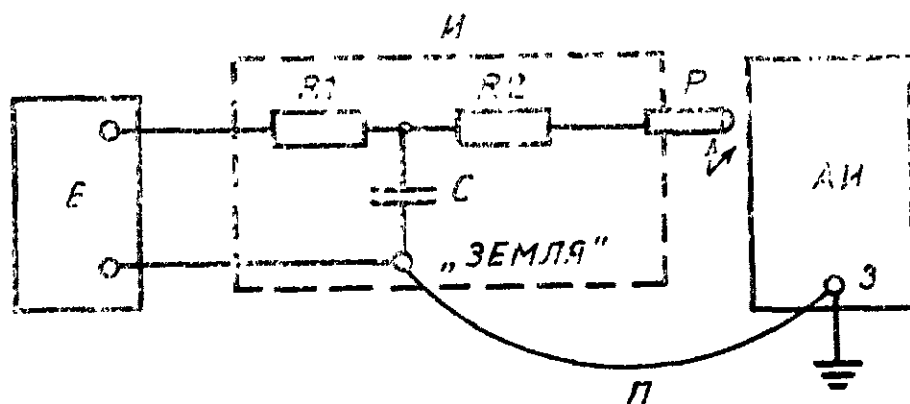
Схема соединений испытуемого автомата и прибора при испытаниях по п. 1.1.4
