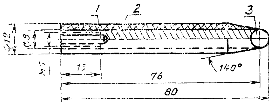
Разрядный наконечник имитатора
