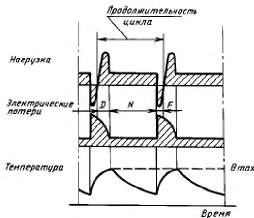
Периодический непрерывный режим с электрическим торможением Типовой режим S7
