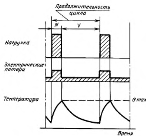
Периодический непрерывный режим с кратковременной нагрузкой Типовой режим S6
