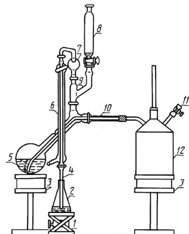
1 — подъемный столик; 2 — приемная колба; 3 — нагревательное устройство; 4 — удлиненная муфта; 5 — отгонная колба; 6 — холодильник; 7 — каплеуловитель; 8 — делительная воронка; 9 — переход; 10 — изоляция паропроводящей трубки; 11 — отвод с зажимом; 12 — парогенератор
