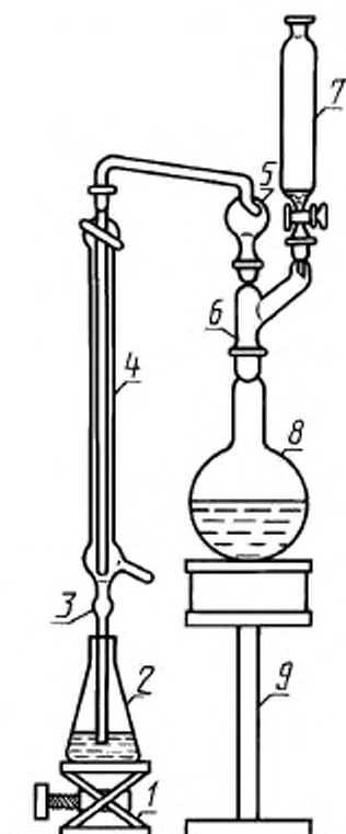
1 — подъемный столик; 2 — приемная колба; 3 — удлиненная муфта; 4 — холодильник; 5 — каплеуловитель; 6 — переход; 7 — делительная воронка; 8 — отгонная колба; 9 — нагревательное устройство
