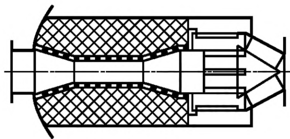
е) Глушитель с искрогасителем
