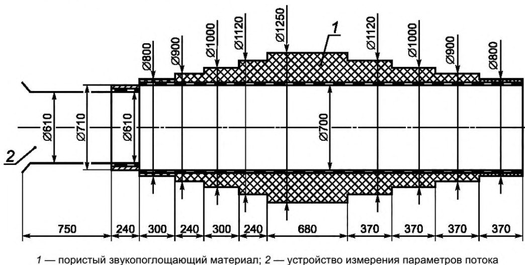
Рисунок G.1 — Пример концевого поглощающего устройства
