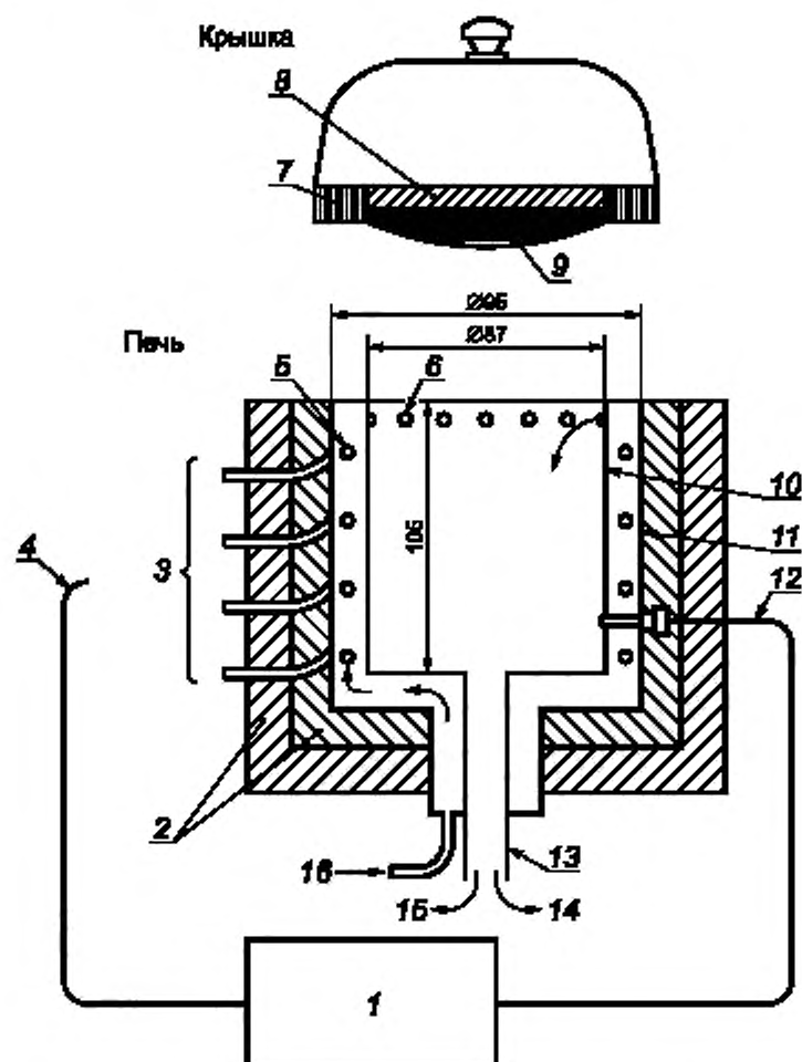
1 — микропроцессорный контроллер; 2 — 2 слоя изоляции; 3 — 2 обмотки трубчатого нагревателя 700 Вт; 4 — провода нагревателя; 5 — поперечное сечение обмотки нагревателя; 6 — 2 отверстия диаметром 1 мм; 7 — керамическое кольцо; 8 — изоляция; 9 — верхняя круглая заглушка из нержавеющей стали марки 304; 10 — внутренний цилиндрический кожух из нержавеющей стали марки 304 толщиной 1,6 мм; 11 — наружный цилиндрический кожух из нержавеющей стали марки 304 толщиной 1,6 мм; 12 — провода термопары; 13 — трубка из нержавеющей стали диаметром 13 мм; 14 — конденсат; 15 — дым; 16 — азот
