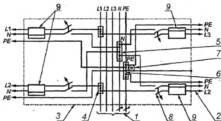
1 – питающая цепь; 2 – распределительная цепь; 3 – проводящая оболочка* щитка; 4, 5, 6 – зажимы для проводников питающей цепи (фазных, нулевых, защитных PE, нулевых рабочих N) и проводников распределительных цепей; 7 – знак заземления у зажимов (позиция 6); 8 – автоматический выключатель; 9 – счетчик
