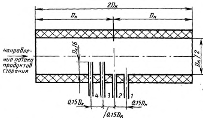
Участок для измерения параметров продуктов сгорания
