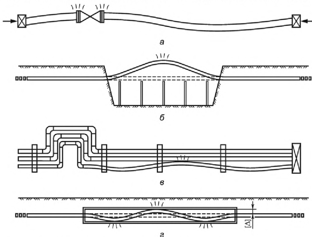
a — форма потери устойчивости трубопровода, б — то же при надземном переходе через реку, в — то же на эстакаде, г — то же в канале
