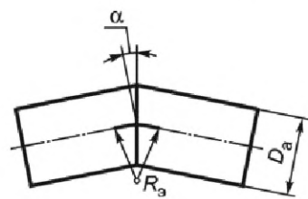
Рисунок 9.2 — Косой стык
