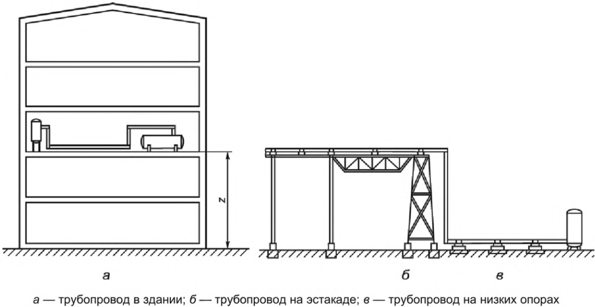
Рисунок 16.1 — Варианты расположения трубопровода
