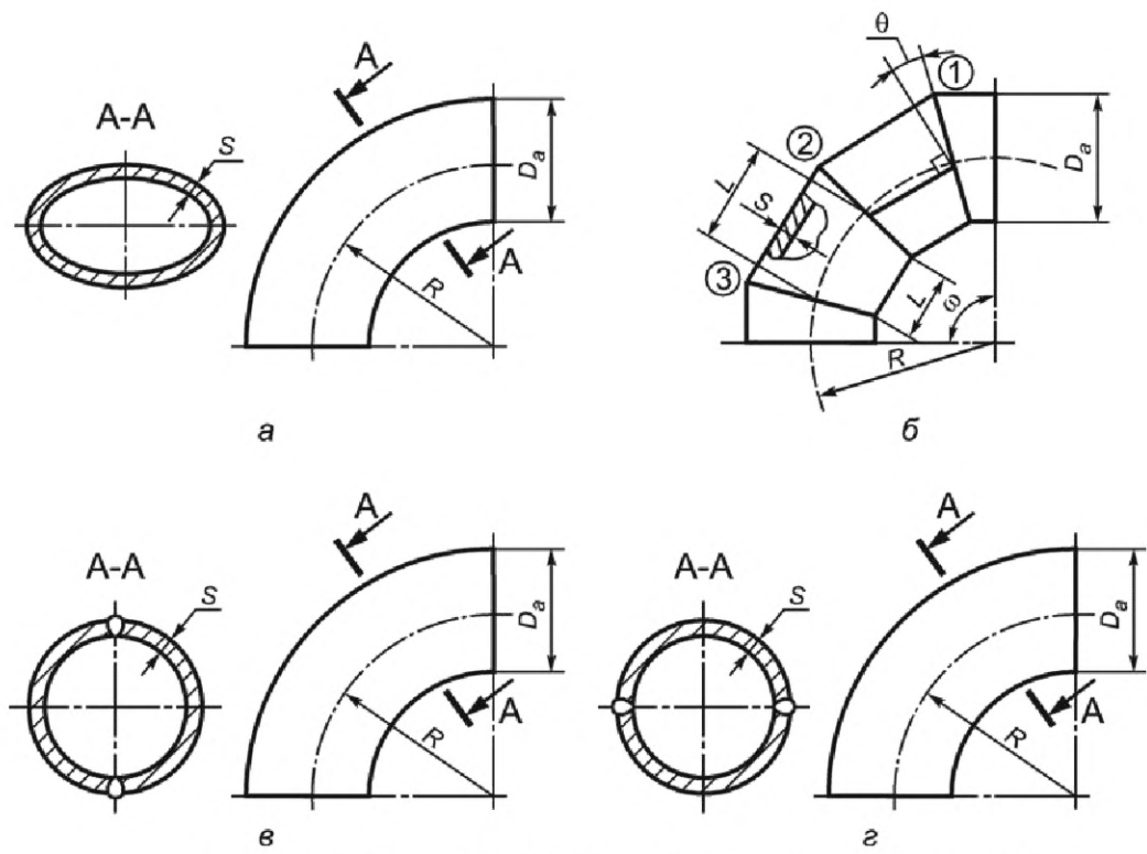
а — гнутый; б — секторный с тремя косыми стыками (n = 3); в и г — штампосварной
