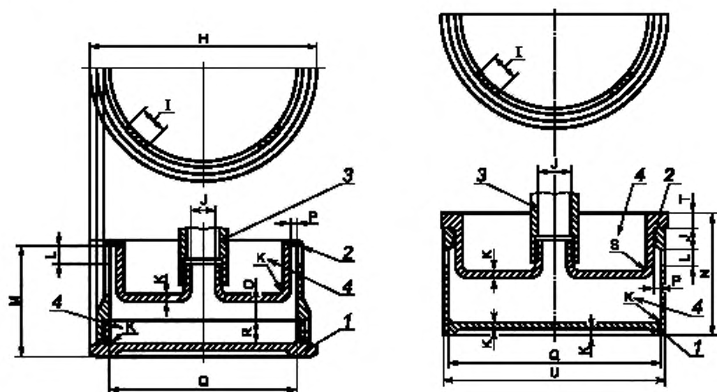
а) Чашка для образца пластинной смазки
