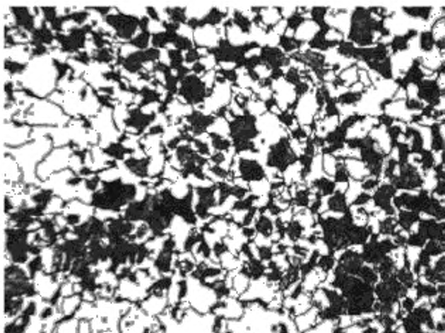
Кратность увеличения 500×
