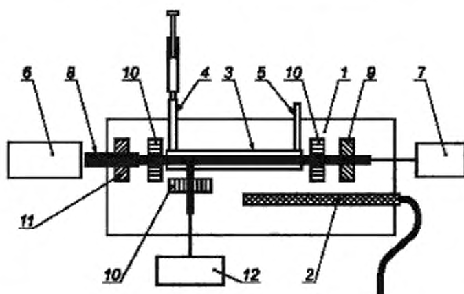
1 — камера для образца; 2 — устройство измерения температуры (датчик); 3 — испытательная ячейка для образца; 4 — входное отверстие для образца; 5 — выходное отверстие для образца; 6 — лазер; 7 — детектор кристаллов (см. кривую сплошной линией на рисунке А1.3 приложения А1); 8 — оптический контур; 9 и 11 — поляризационные фильтры; 10 — окошки; 12 — детектор помутнения (см. кривую пунктирной линией на рисунке А1.3 приложения А1)
