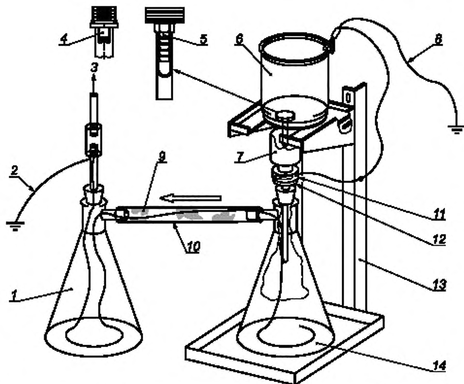
1 — толстостенная колба; 2 — лабораторное заземление (обычное); 3 — к вакуумному насосу; 4 — раздаточная пробка; 5 — раздаточный коппачок с резьбой; 6 — контейнер для образца; 7 — фильтрующая воронка; 8 — провод заземления; 9 — уплотняющий материал между трубкой, шлангом и проводом; 10 — резиновый вакуумный шланг; 11 — стопорное кольцо; 12 — основание мембранного фильтра; 13 — штатив; 14 — приемная колба
