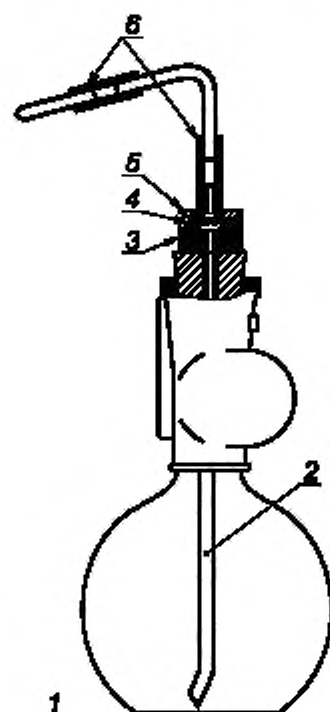
1 — устройство для фильтрования растворителя, 2 — пластиковая трубка из материала, стойкого к растворителям, 3 — опорное кольцо из инертного материала, 4 — мембранный фильтр с размером пор 0,45 мкм, 5 — опорное кольцо из инертного материала, 6 — пластиковое соединение из материала, стойкого к воздействию реактивов
