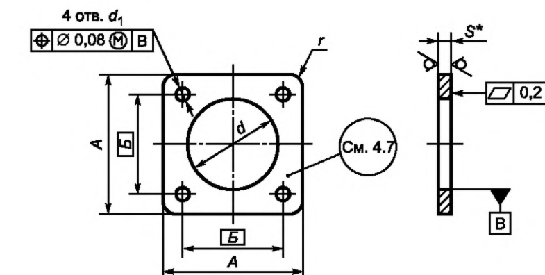
Рисунок 2 — Держатель ДП
