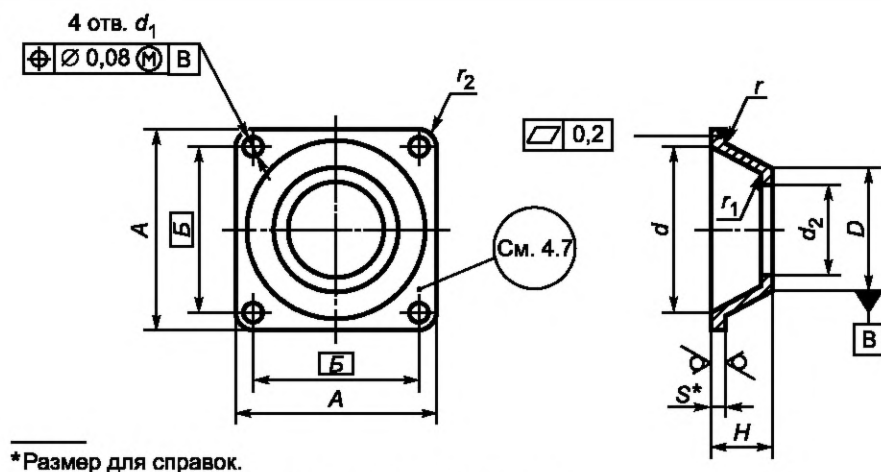
Рисунок 3 — Держатель ДЧ
