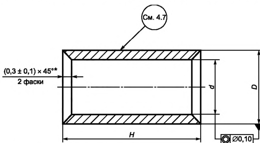
Рисунок 1 — Конструкция втулок
