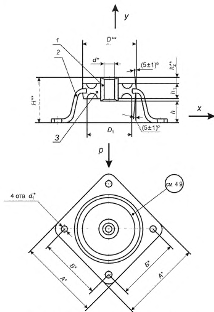
Рисунок 2 — Амортизатор типа АЧ
