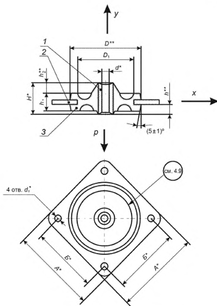
Рисунок 1 — Амортизатор типа АП
