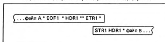
Пустая секция файла в промежуточном конце дорожки
