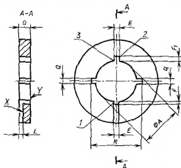
Калибр для проверки крепления цоколей типов В15d и В22d в патроне
