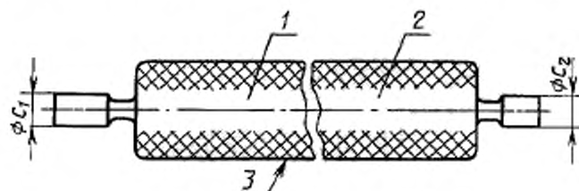
1 — проходной калибр; 2 — непроходной калибр; 3 — накатка
