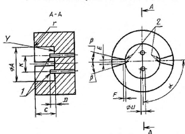
Калибр для проверки цоколей типа В22d, предназначенных для автоматической установки токовых вводов ламп
