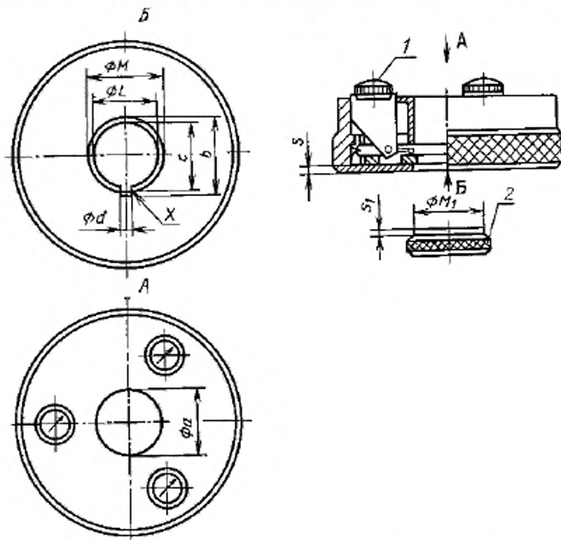
1 — регулирующий циферблатный индикатор; 2 — блок регулирующего устройства
