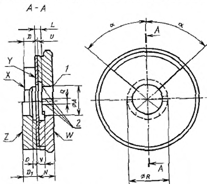
Проходной калибр для проверки цоколя типа BAY—15d на готовой лампе
