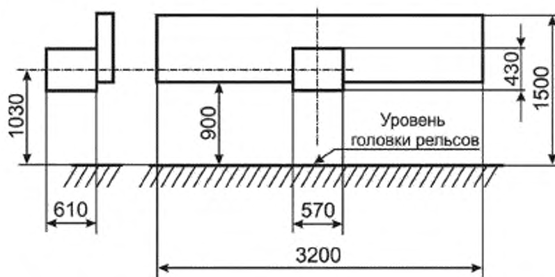
Рисунок 2 — Размеры препятствия при аварийном столкновении по сценарию 2
