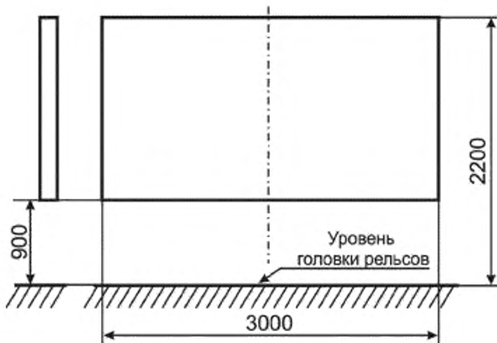
Рисунок 1 — Размеры препятствия при аварийном столкновении по сценарию 1
