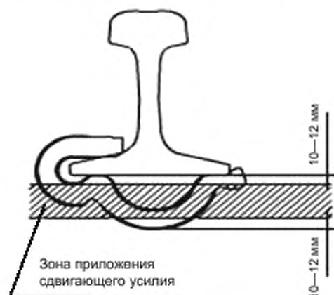
Рисунок 4 — Схема проверки удерживающей способности противоугона для железнодорожного пути на деревянных шпалах
