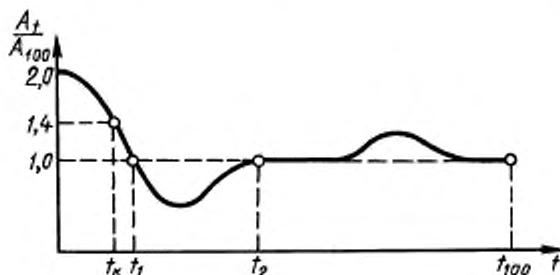
Влияние положительного наложения между t_2 и t_{100}
