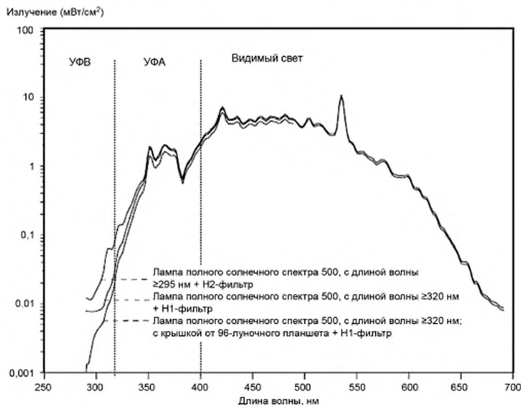
Рисунок 1 — Спектральное распределение излучения солнечного имитатора
