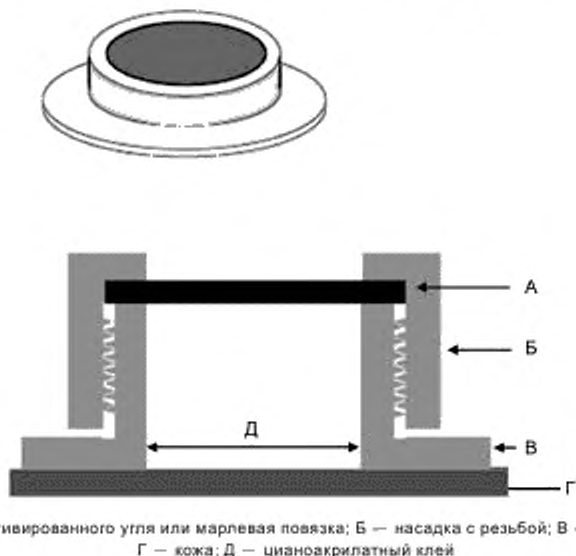
Рисунок 1 — Пример стандартного устройства, используемого для ограничения и защиты места нанесения вещества во время исследований перкутанной абсорбции in vivo
