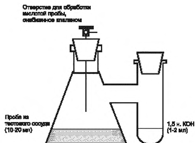
Рисунок А.3 — Система для улавливания растворенного ^{14}\text{CO}_2
