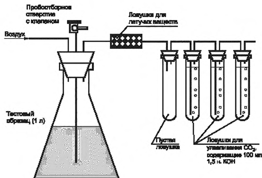
Рисунок А.1 — Пример проточной испытательной установки
