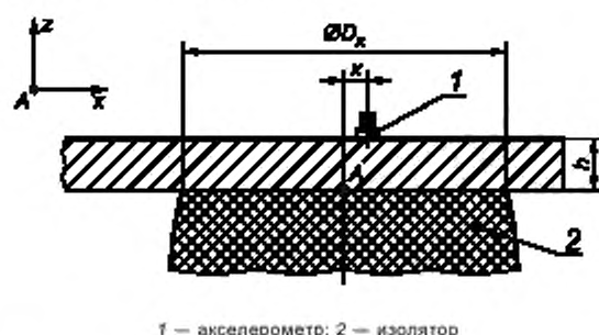
Рисунок 4 — Положение акселерометра для измерений v_z
