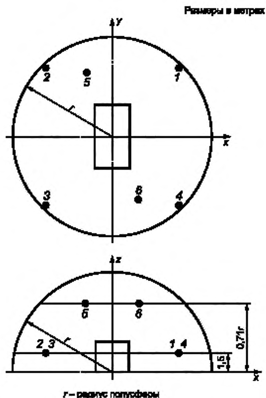
Рисунок 1 — Положения микрофонов на полусфере (см. таблицу 2)
