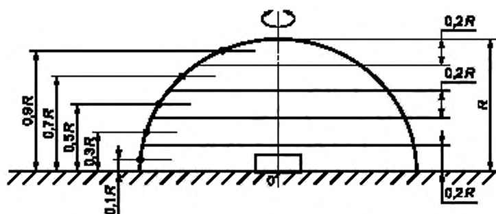
Рисунок А.2 — Соосные круговые траектории микрофона
